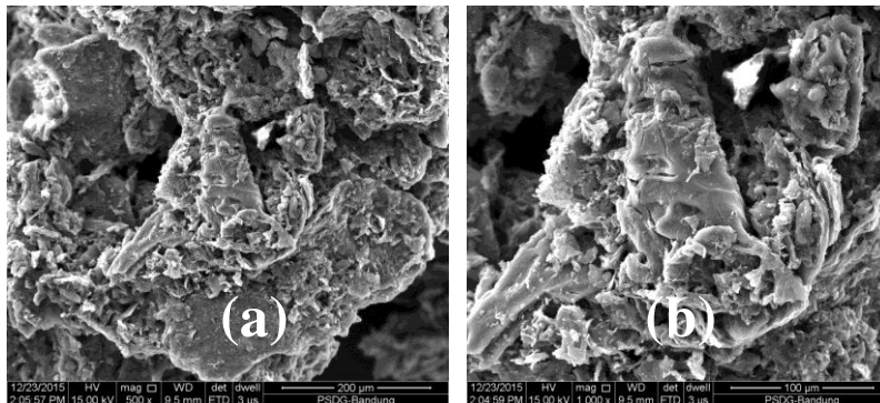
Gambar 2 Hasil SEM EDS Karbon Aktif (a) 500 kali (b) 1000 kali
