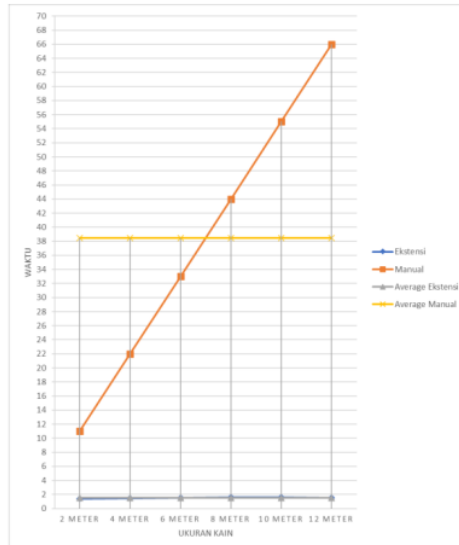
Gambar 13. Grafik waktu pembuatan program CNC
