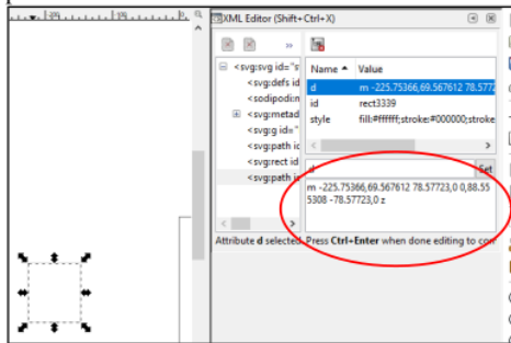
Gambar 2. Model matematis sebuah gambar pada software inkscape
