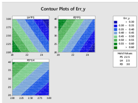
Gambar 7. Contour plots respon error dimensi y
