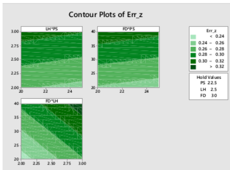
Gambar 8. Contour plots respon error dimensi z
