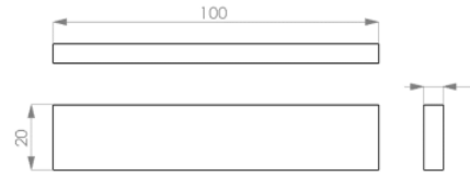
Gambar 3. Dimensi spesimen
