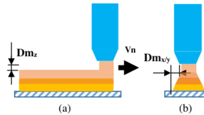
Gambar 12. Skema visualisasi printing
