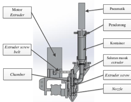
Gambar 2. Sistem ekstruksi
