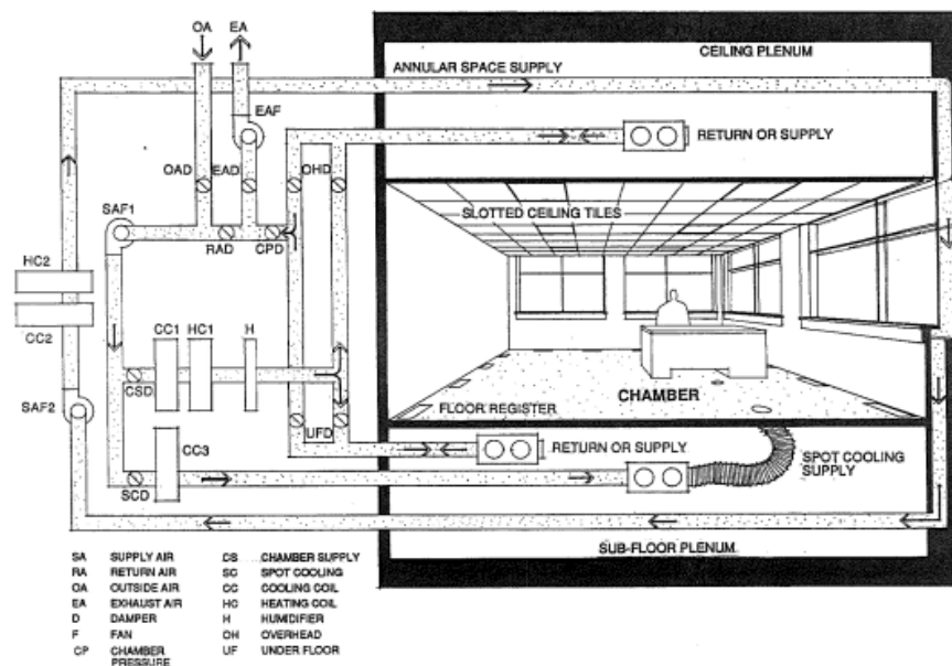
Gambar 8. Sistem pengatur sirkulasi udara yang menjadi fasilitas suatu ruang (Sumber: Baumen dan Arens, 1988)
