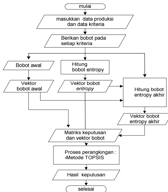
Gambar 4. Proses pemilihan subkontrak
