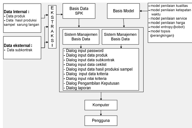
Gambar 1. Komponen sistem pendukung keputusan pemilihan subkontrak
