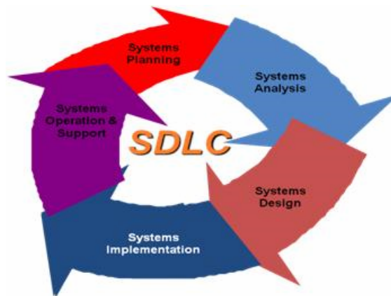
Gambar 3. Tahapan SDLC
