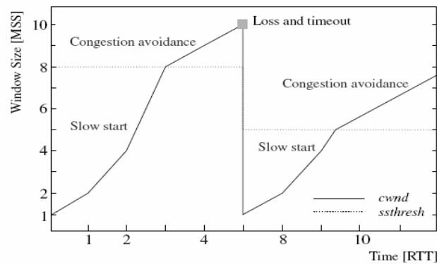
Gambar 2.1 Ilustrasi Ukuran W pada TCP reno
