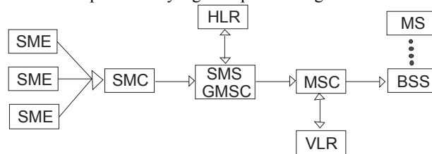
Gambar 2. Elemen Jaringan dan Arsitektur SMS
