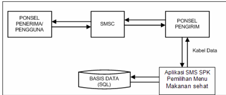
Gambar 5. Arsitektur Sistem
