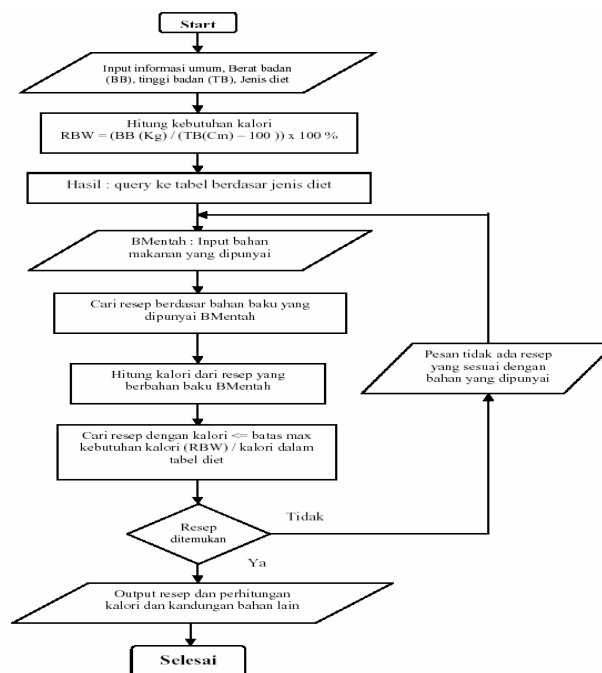
Gambar 4. Diagram alir proses sistem
