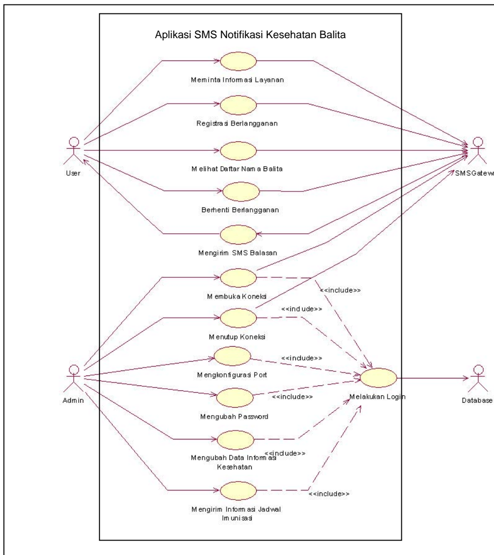
Gambar 1. Diagram Use Case Aplikasi SMS Notifikasi Kesehatan Balita
