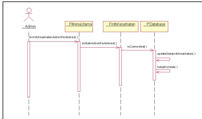
Gambar 7. Diagram Sequence Mengubah Data Informasi Kesehatan
