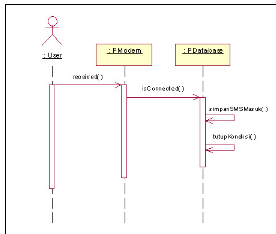
Gambar 4. Diagram Sequence Melihat Daftar Nama Balita
