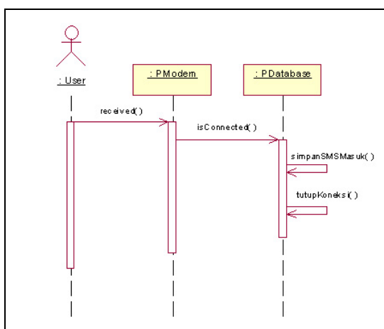
Gambar 2. Diagram Sequence Meminta Informasi
