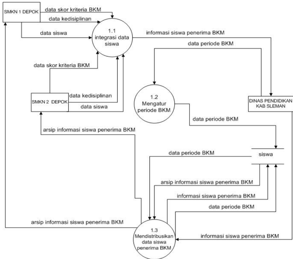
Gambar 2. DFD Level 1
