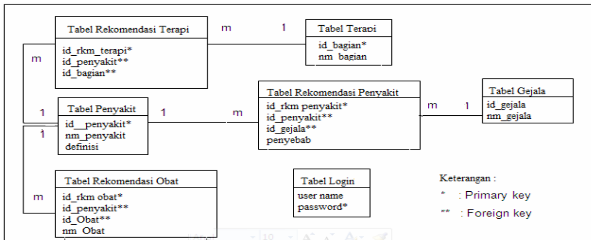
Gambar 3. Relasi Antar Tabel
