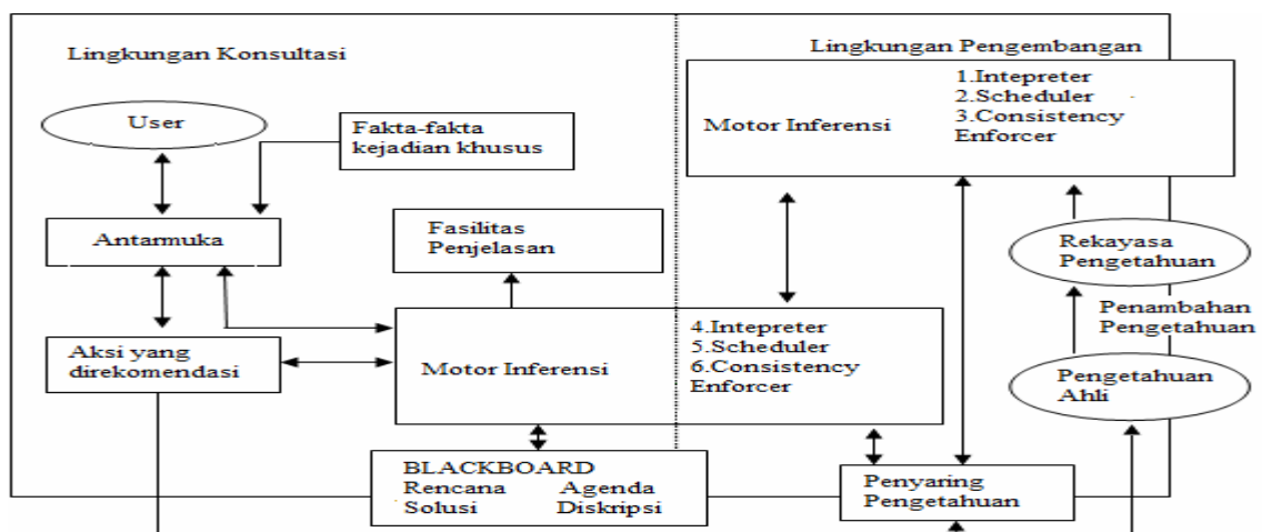
Gambar 1. Struktur Sistem Pakar.
