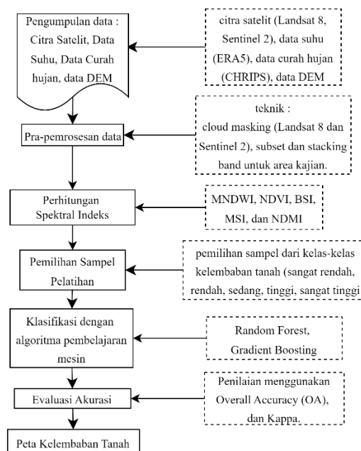
Gambar 1. Metode Penelitian Pemodelan Spasial Kelembaban Tanah
