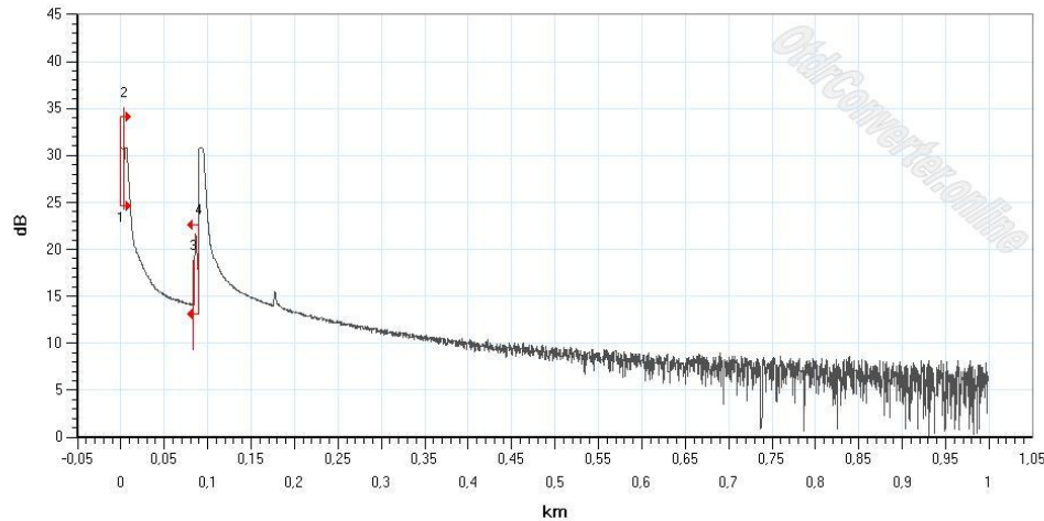
Gambar 4.1 Hasil Pengukuran OTDR
