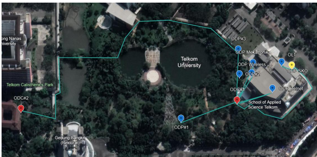
Gambar 3.2 Desain Pergelaran Jaringan Fiber Optik
