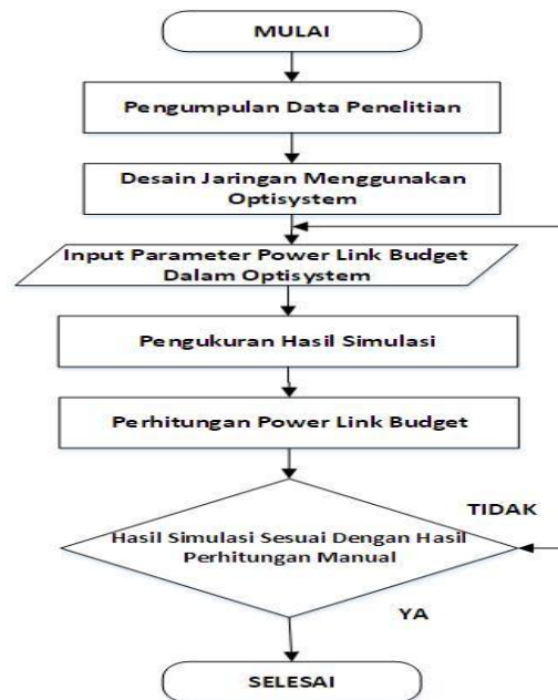
Gambar 3.1 Diagram Alir
